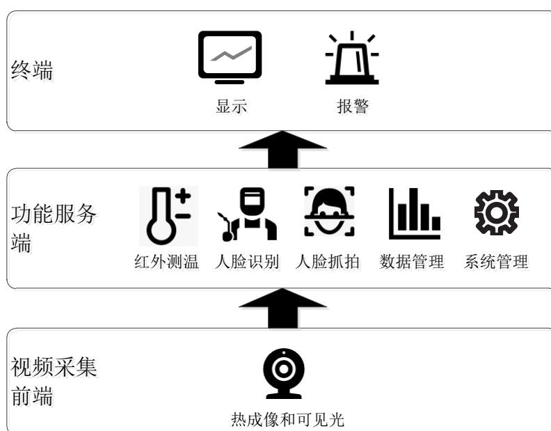
图1 热成像人体测温报警系统架构
